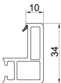
80034 - Зажимной профиль 10мм х 34мм
