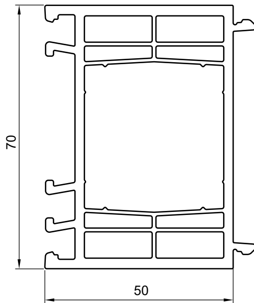
Расширитель «50» 57056
