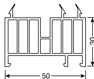
Монтажный профиль 68071
