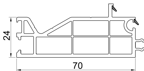
80070 - Базовый профиль 24мм х 70мм
