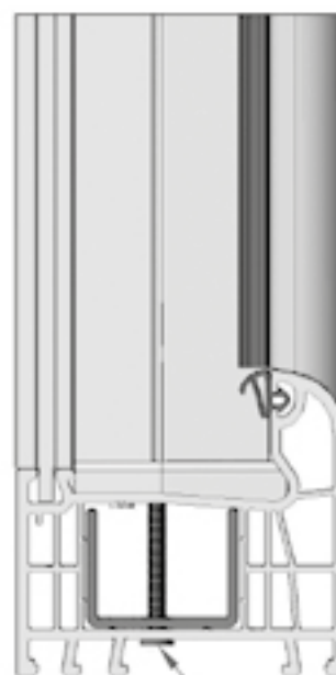
боковой вид
