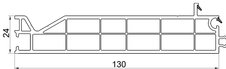
80130 - Базовый профиль 24мм х 130мм
