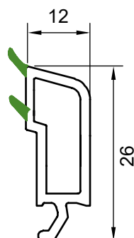
штапик 68644 Стеклопакет 48 mm
